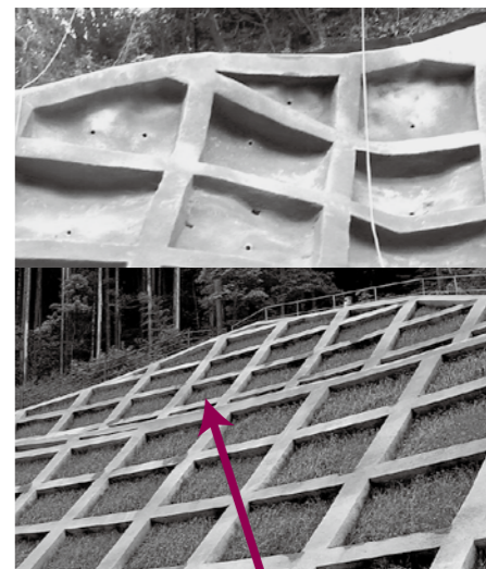
法砕工による復旧イメージ
