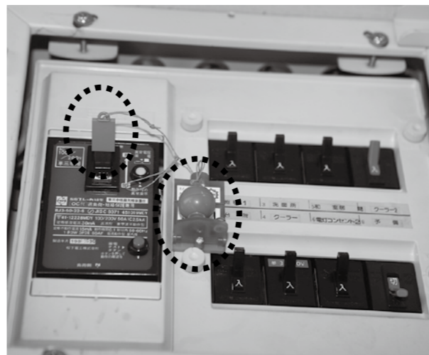
地震時の電気火災を抑制する感震ブレーカー（点線で囲った部分）
